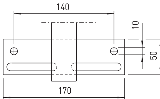
SCD, fodplade til SE150 ben, set ovenfra
